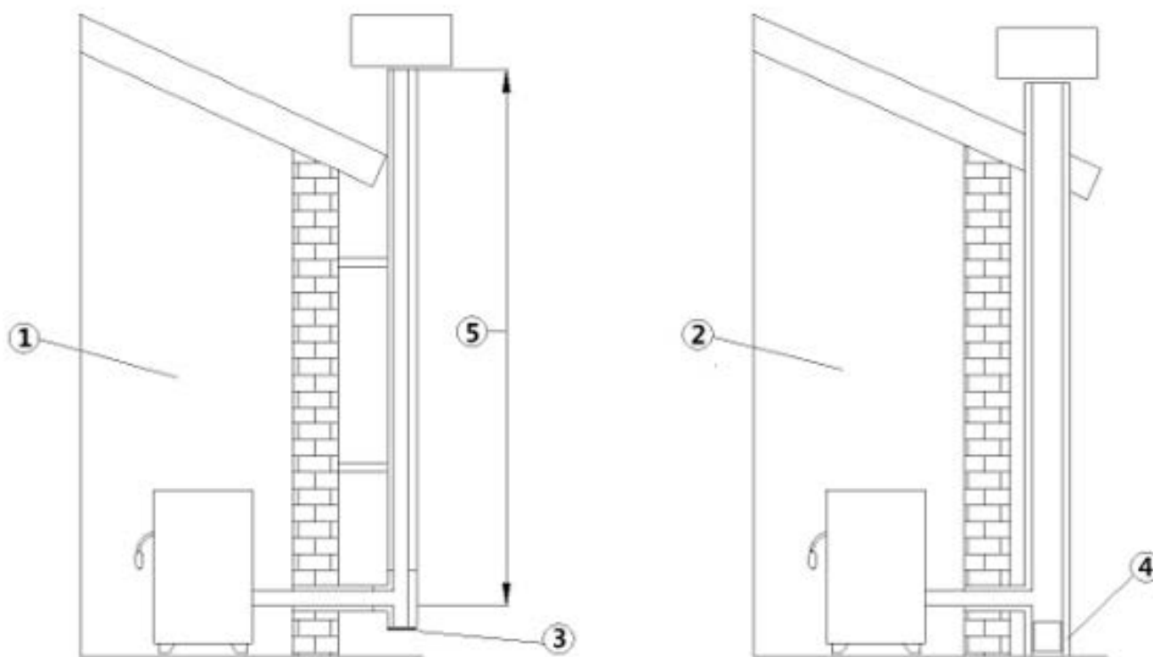
Fig. 3 - Canne fumarie
