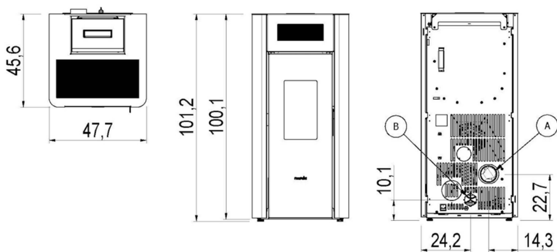
Fig. 18 - Dimensioni generali: Amaranato 9
