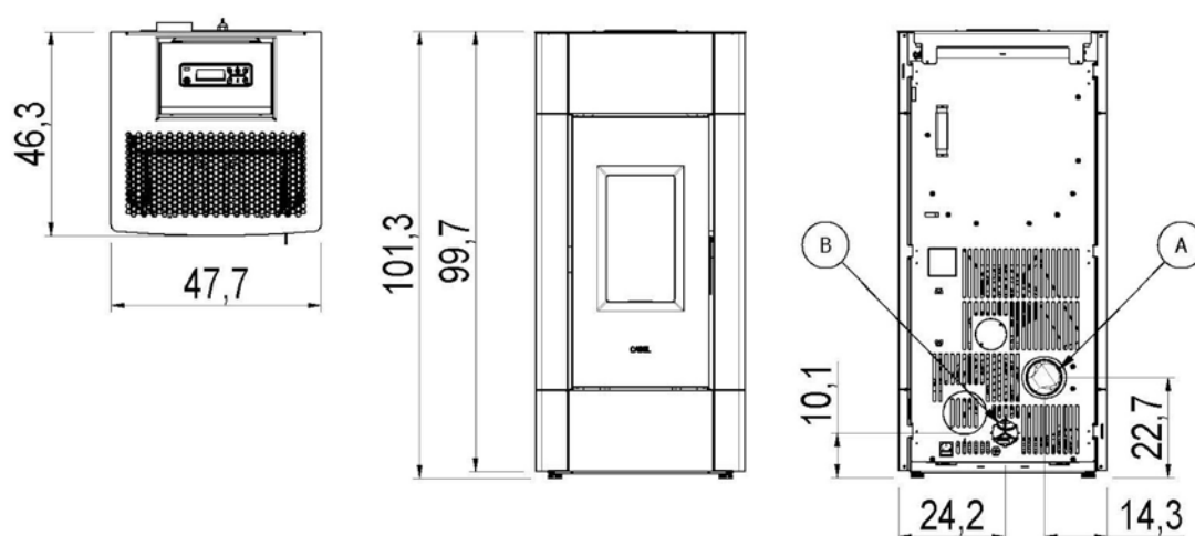
Fig. 15 - Dimensioni generali: Cristal 9
