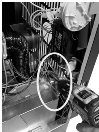
Fig. 60 - Bloccare tubo flessibile
