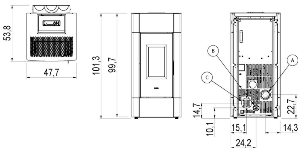
Fig. 16 - Dimensioni generali: Cristal Plus 9
