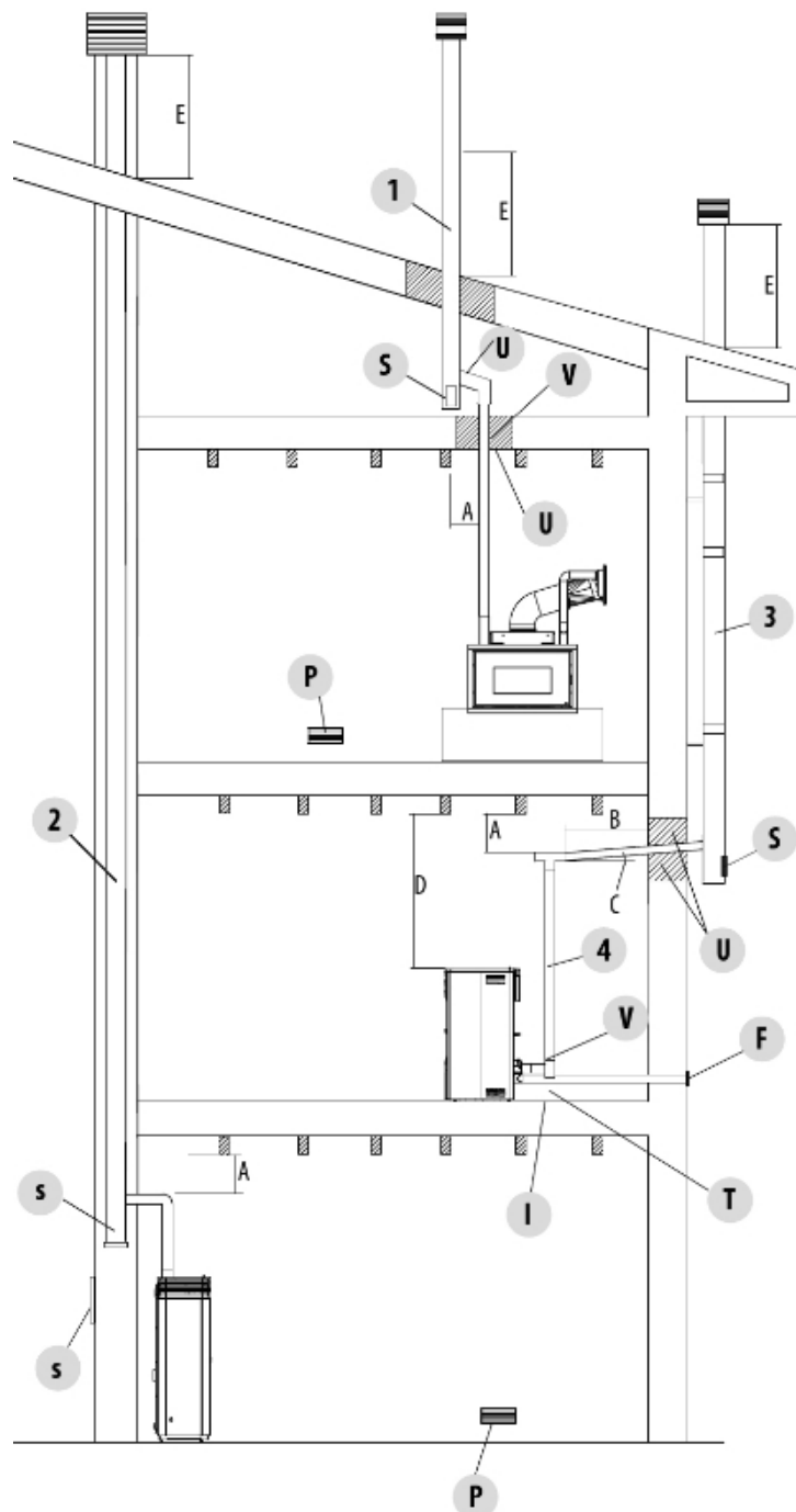
Fig. 13 - Canna fumaria
