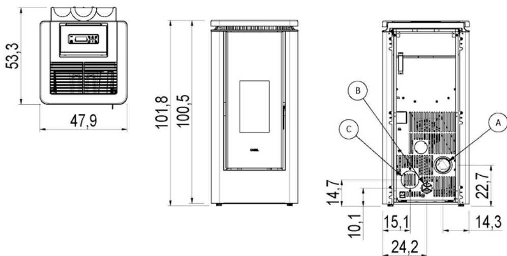
Fig. 17 - Dimensioni generali: Icon Plus 9
