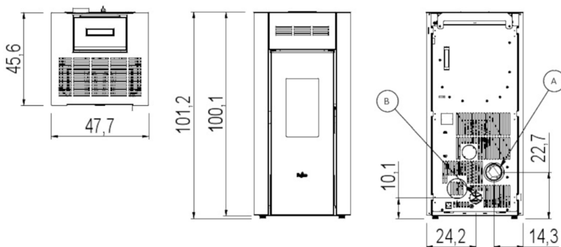
Fig. 21 - Dimensioni generali: Elane 9
