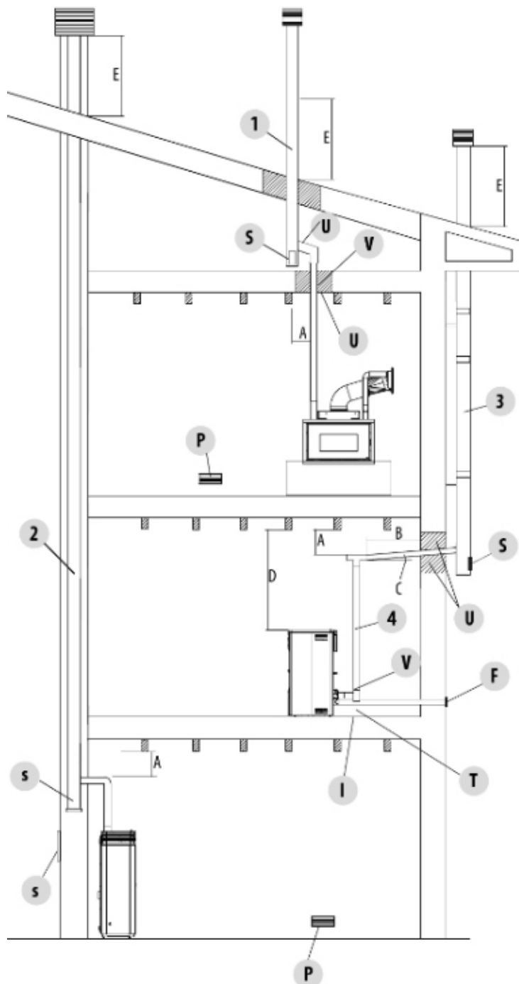
Fig. 10 - Canna fumaria
