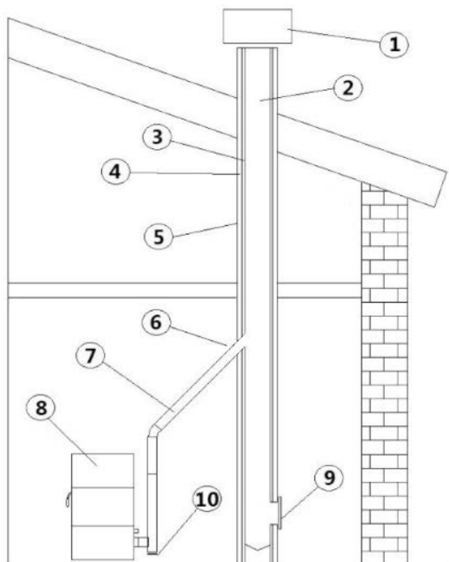
Fig. 2 - Componenti camino
