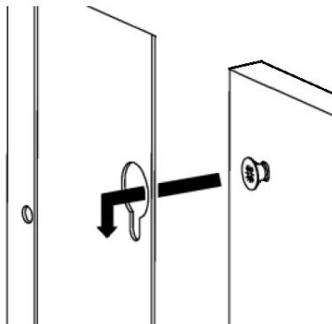
Fig. 61 - Dettaglio dell'aggancio
