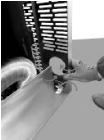
Fig. 90 - Piegare le linguette
