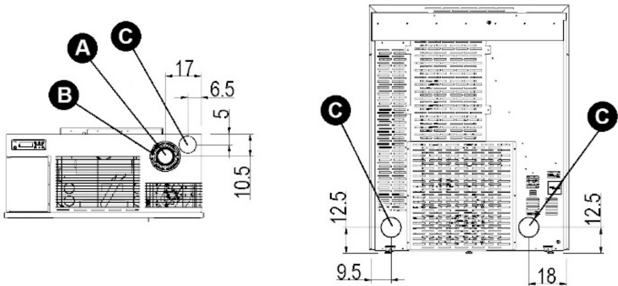
Fig. 16 - Dimensioni generali: Mithos3 Plus 12/14
