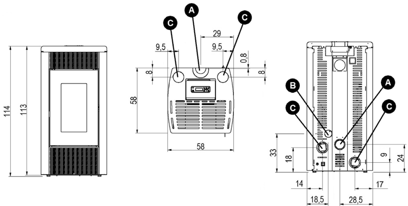
Fig. 13 - Dimensioni generali: Duke 12/14 Airtight
