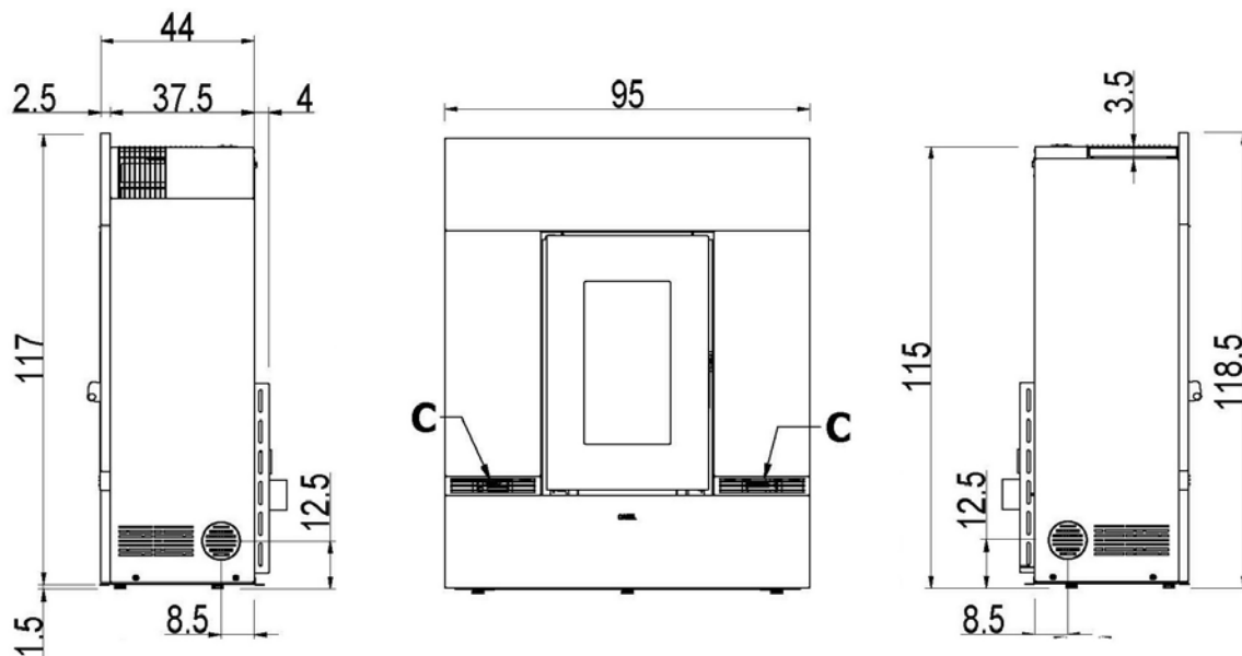
Fig. 17 - Dimensioni generali: Mithos Plus 12/14 PS
