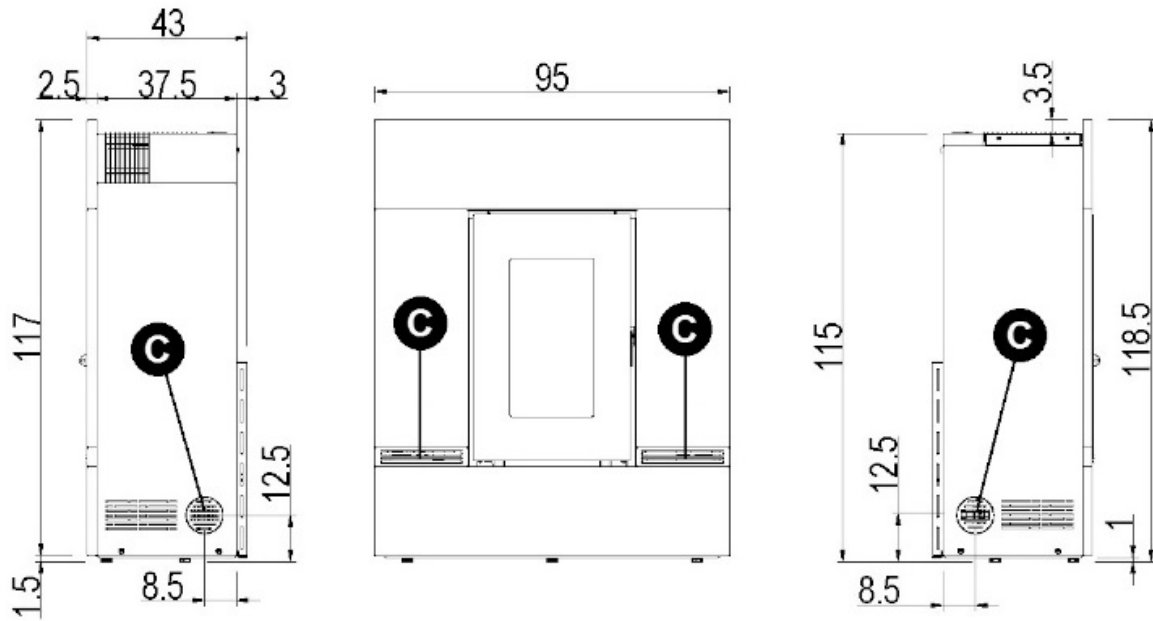
Fig. 15 - Dimensioni generali: Mithos3 Plus 12/14
