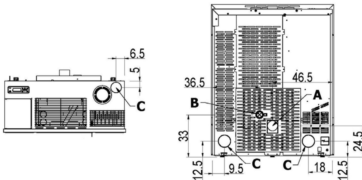
Fig. 18 - Dimensioni generali: Mithos Plus 12/14 PS
