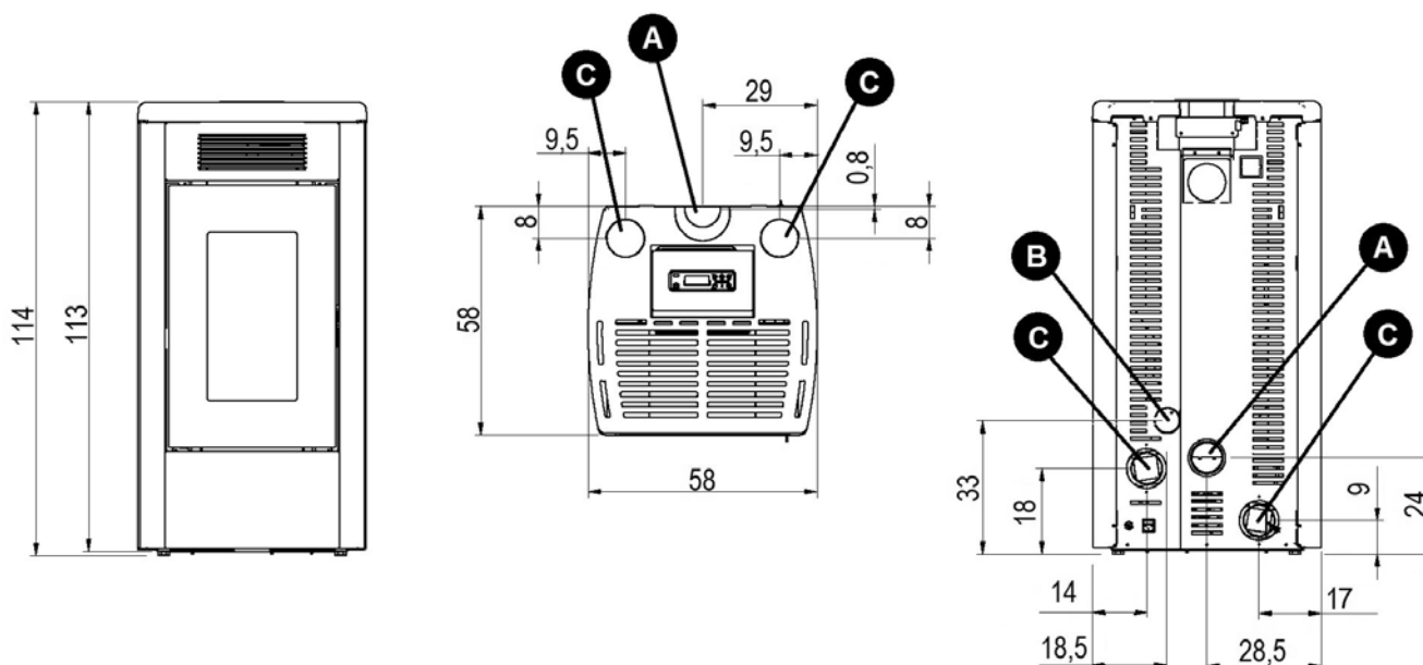
Fig. 12 - Dimensioni generali: Atena³ Plus 12/14
