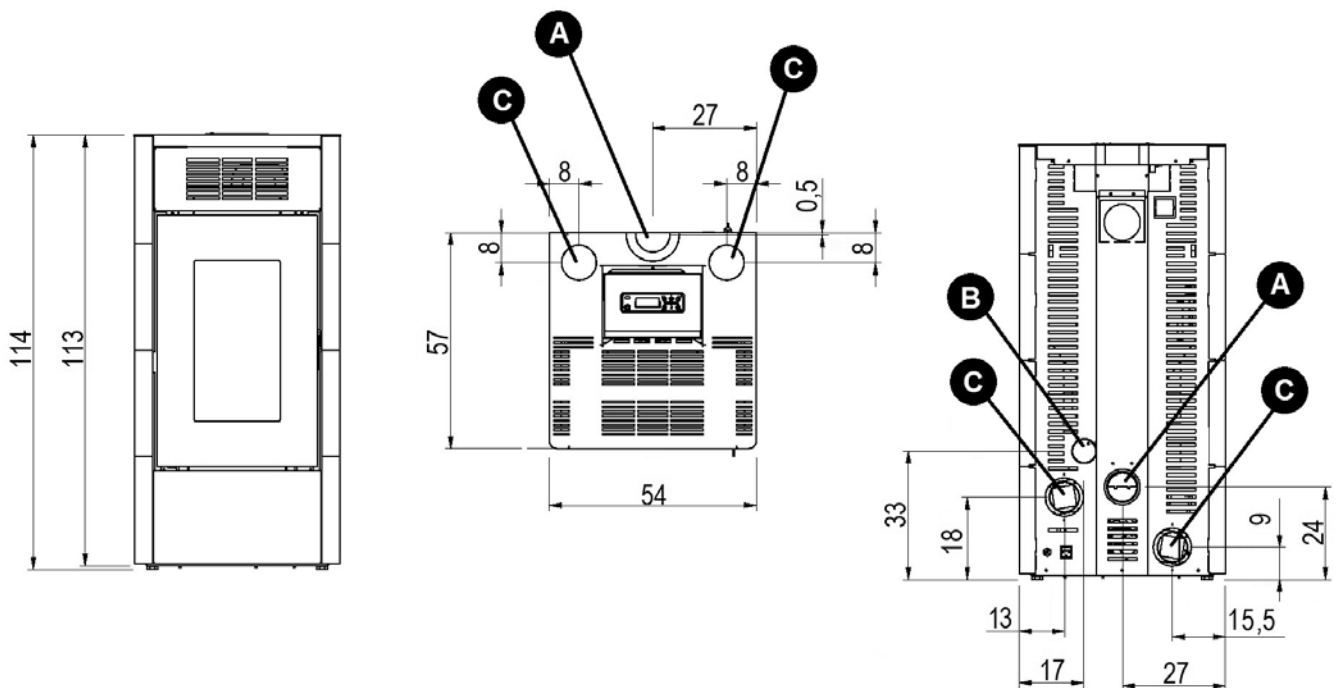
Fig. 14 - Dimensioni generali: Saba 12/14
