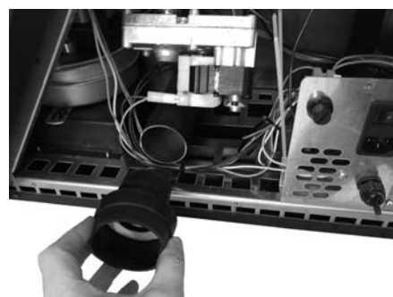
Fig. 43 - Rimuovere raccordo siliconico
