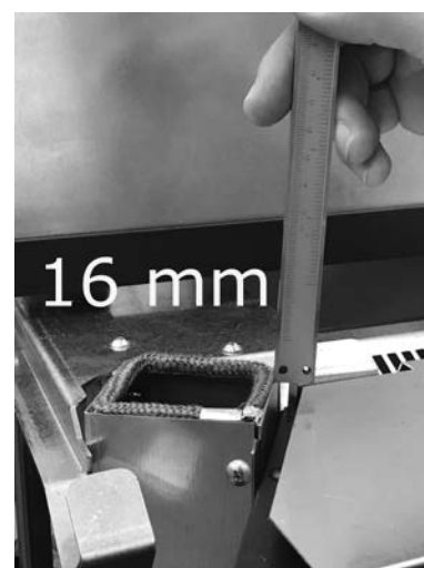
Fig. 42 - Sporgenza del deviatore aria
