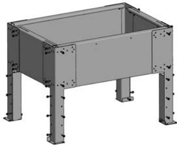
Fig. 30 - Assemblare gambe
