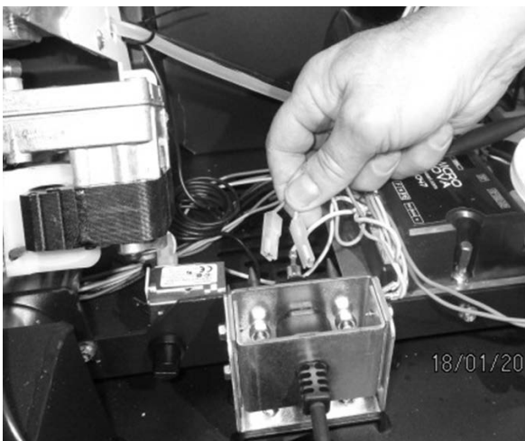
Fig. 83 - Disconnessione faston (blu - marrone)
