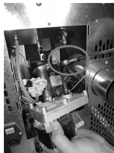
Fig. 88 - Rimozione motoriduttore
