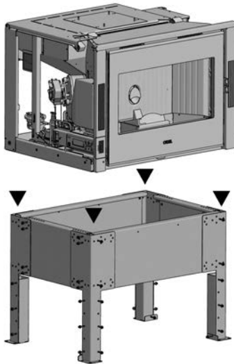
Fig. 32 - Fissare inserto sopra
