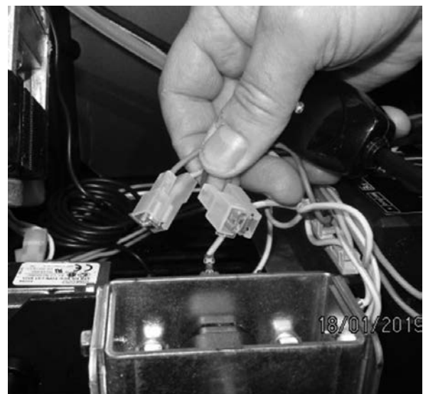
Fig. 84 - Collegamento faston doppi
