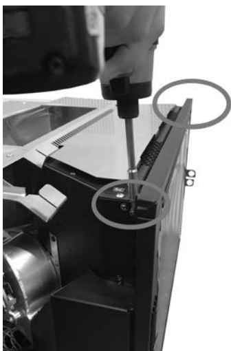
Fig. 47 - Rimozione profilo superiore
