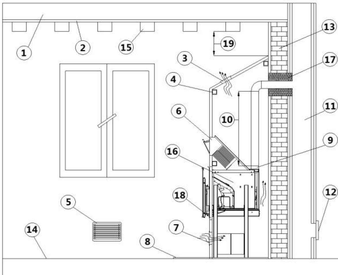
Fig. 22 - Installazione con rivestimento
