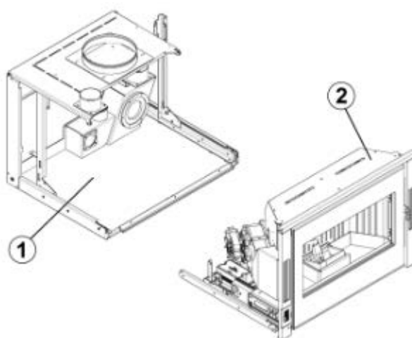
Fig. 15 - Struttura + corpo macchina
