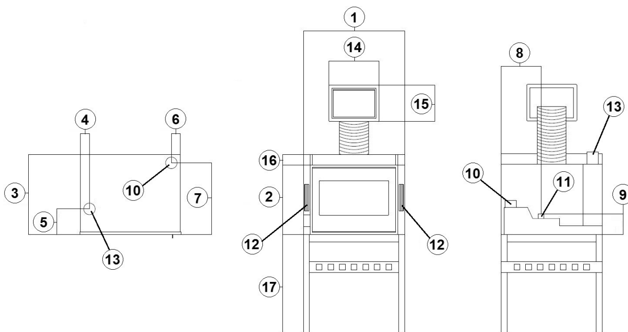
Fig. 14 - Dimensioni generali: Zefiro 3 , Zen Airtight
