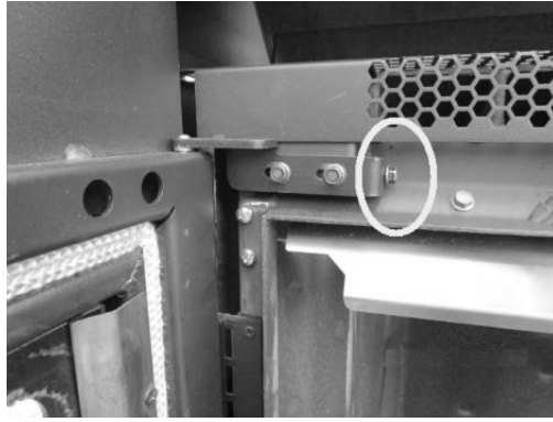
Fig. 24 - Regolazione porta
