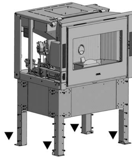
Fig. 33 - Fissare la struttura al pavimento e muro
