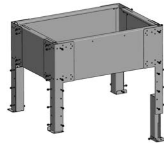
Fig. 31 - Assemblare gambe + prolunga
