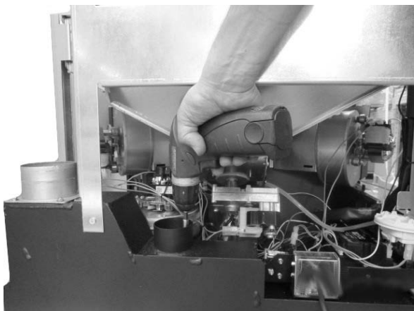
Fig. 28 - Rimozione anello 1
