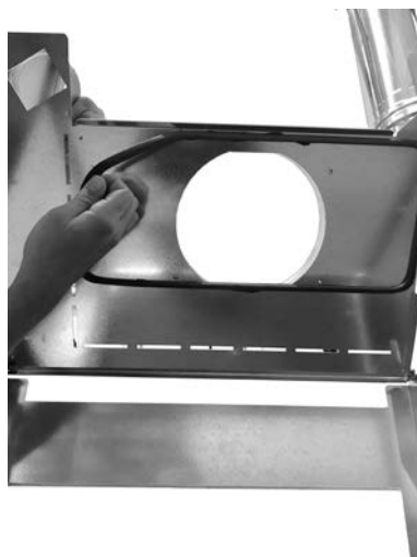
Fig. 48 - Rimozione guarnizione
