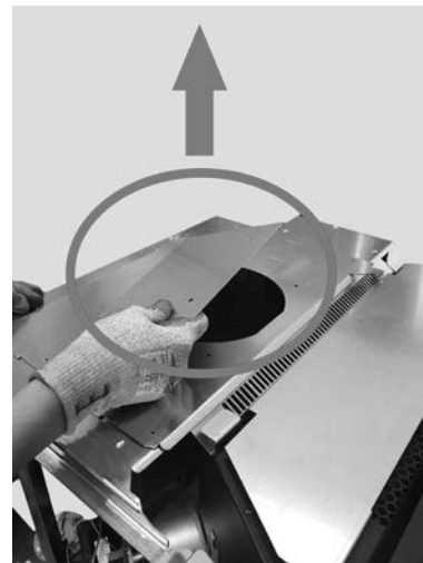
Fig. 60 - Rimuovere tappo
