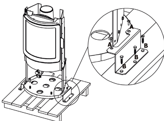
FIG. 4 - RIMOZIONE VITI IMBALLO
