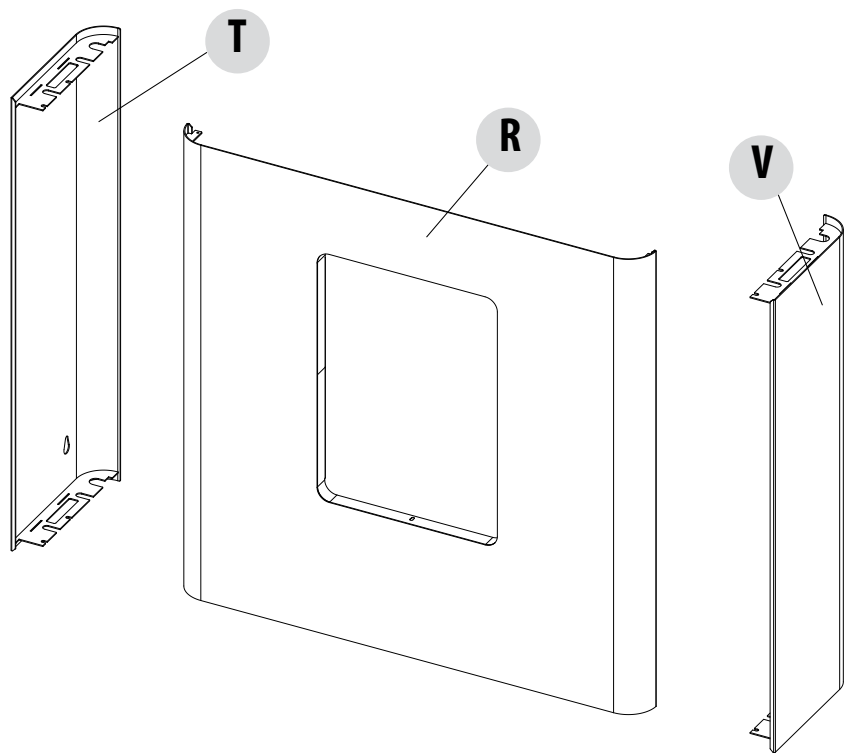
RIVESTIMENTO STUFA
