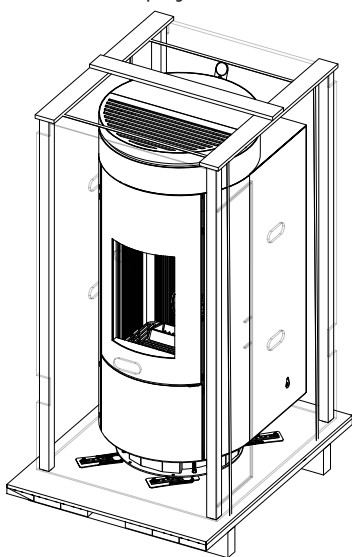
IMBALLO STRUTTURA STUFA
