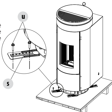
RIMOZIONE STAFFE DI FISSAGGIO
