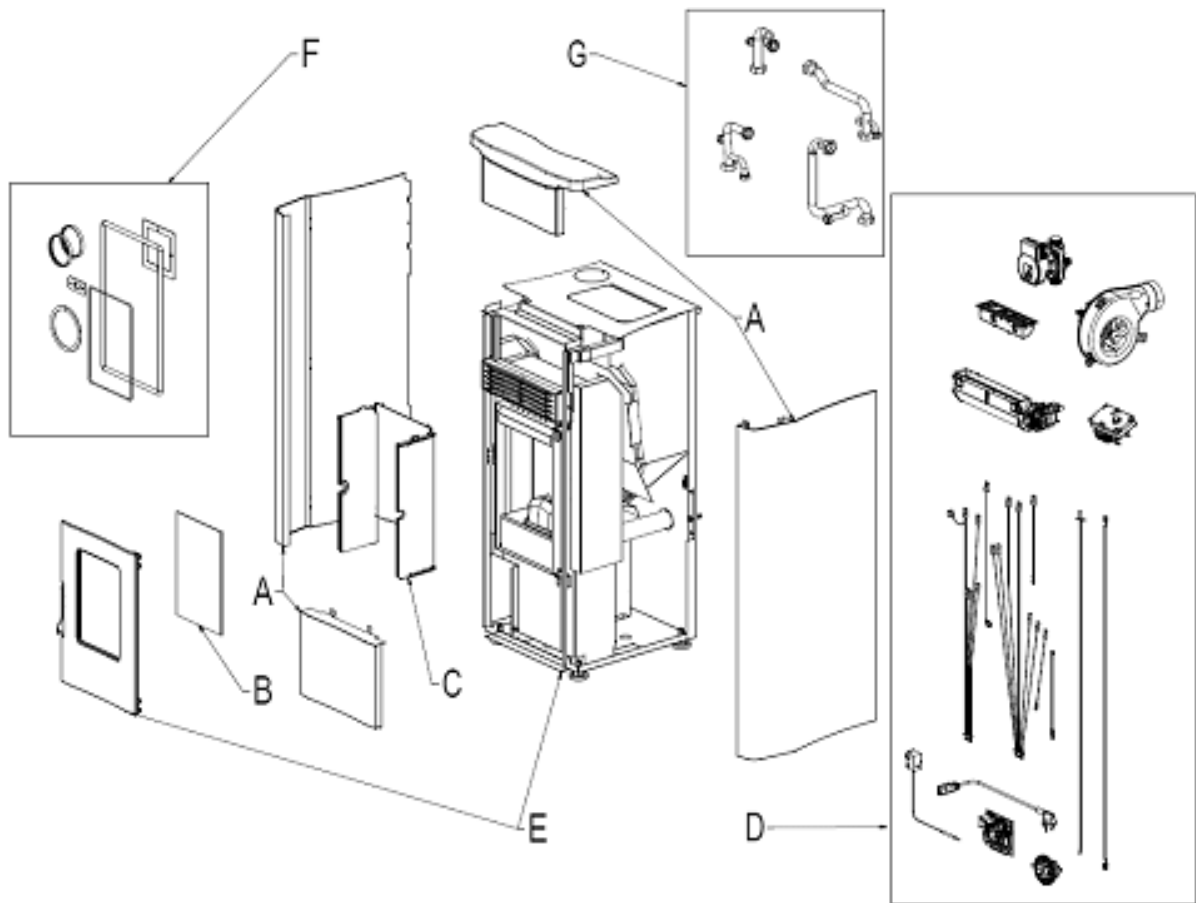
Fig. 1 - Esploso
