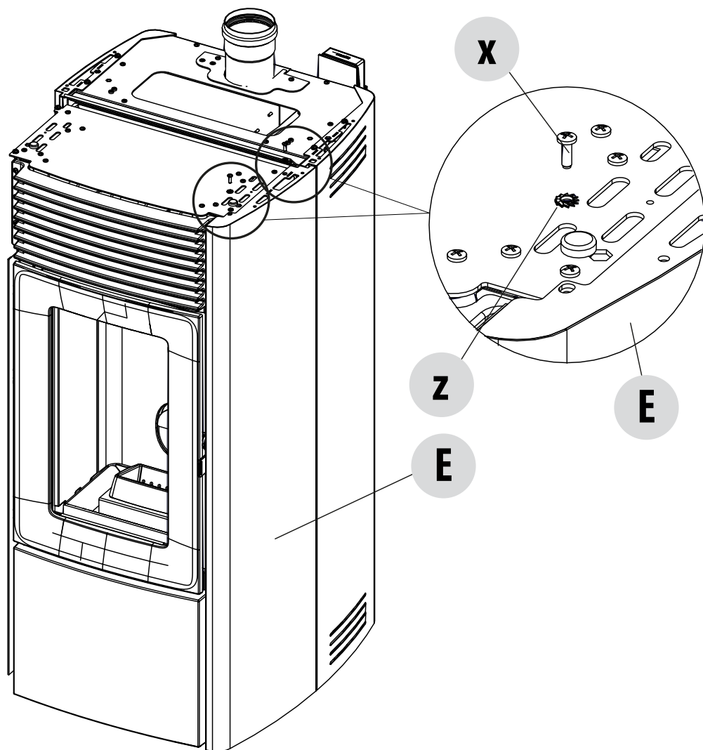
FISSAGGIO SUPERIORE DEL PANNELLO IN METALLO
