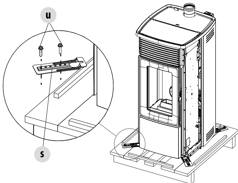
RIMOZIONE STAFFE DI FISSAGGIO (IN FIGURA STUFA EGO)
