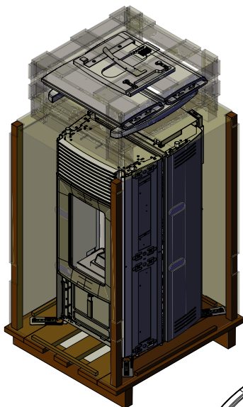
IMBALLO STAR CON RIVESTIMENTO IN CERAMICA (SOPRA)
