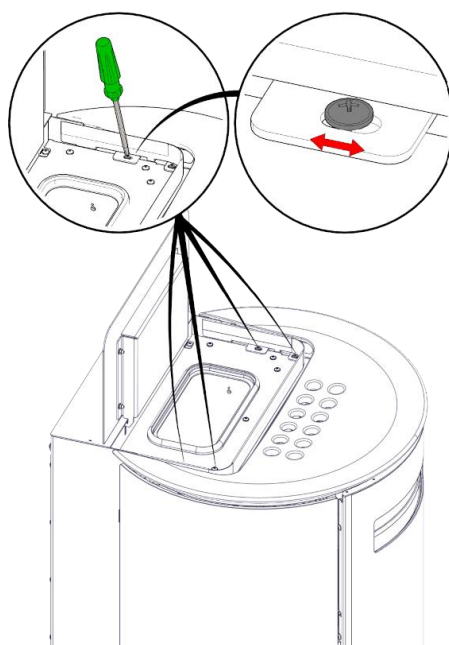
Possibili regolazioni
