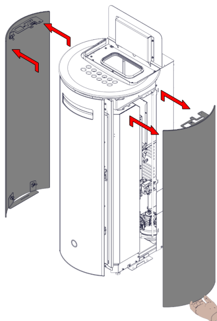
2) Smontare i fianchi
