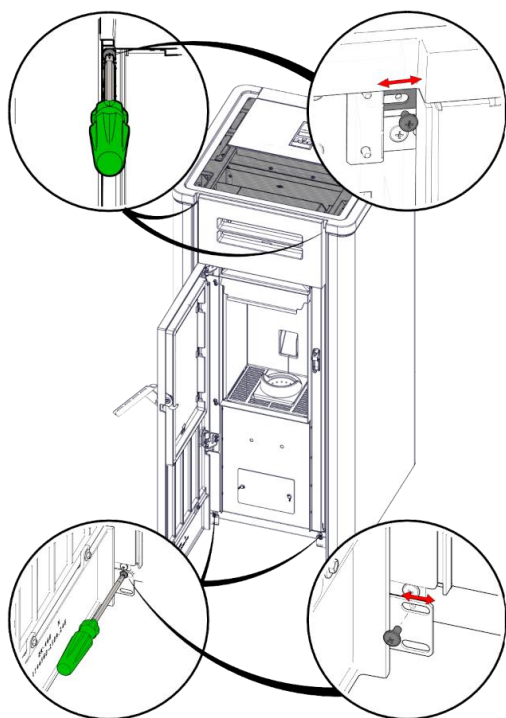
Possibili regolazioni
